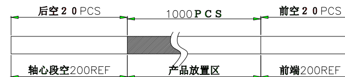
包装示意图:
