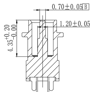
截面A-A
