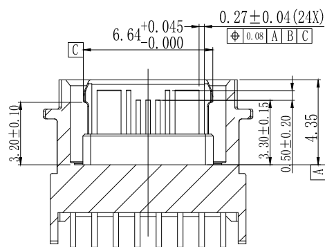
截面B-B
