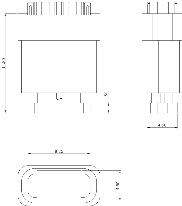
COVER示意图
