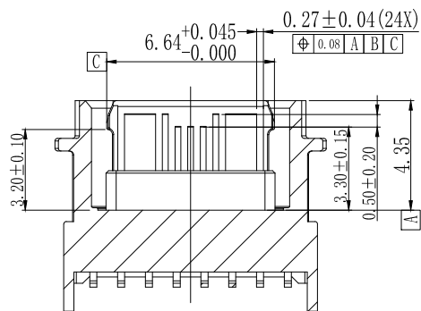
截面B-B
